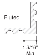
Fig. 2 Ogee Cap & Base PermaWrap® Dimensions*
